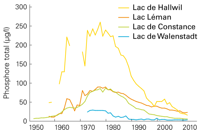
Figure 2: Évolution des teneurs en phosphore dans 4 lacs suisses de 1950 à 2010. En jaune, le lac très eutrophisé de Hallwil, en orange et en vert, les lacs moins affectés du Léman et de Constance et en bleu, le lac peu concerné de Walenstadt. Les apports excessifs de matières nutritives ont des conséquences dramatiques sur les conditions d'oxygénation des profondeurs et peuvent, de ce fait, limiter voire empêcher la reproduction naturelle des salmonidés. Données: OFEV
