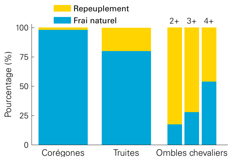
Figure 4: Pourcentage de salmonidés issus du frai naturel (en bleu) ou de repeuplement (en jaune) dans le lac Léman. Les ombles chevaliers ont été répartis en trois classes d'âge (2+, 3+ et 4+). Les poissons de repeuplement de cette espèce ont une plus forte mortalité que leurs congénères nés dans le lac, ce qui explique que leur part relative diminue avec le temps. Données: Commission internationale de la pêche dans le Léman.
