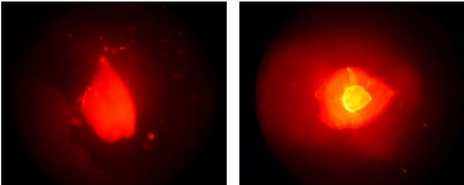
Figure 3: À gauche, un otolithe non marqué, à droite, un otolithe marqué. Les poissons de repeuplement qui ont absorbé le colorant peuvent être identifiés des années plus tard par simple examen microscopique.
