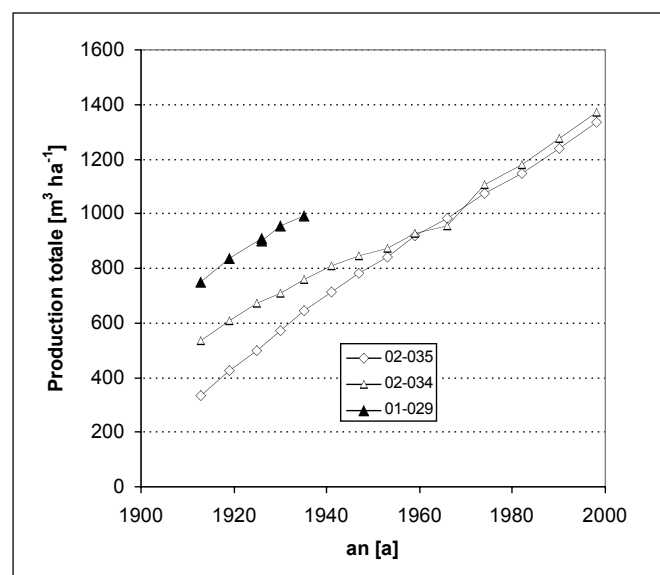
Figure 4: Production totale des parcelles d'essai de forêt jardinée depuis le début de l'essai.
