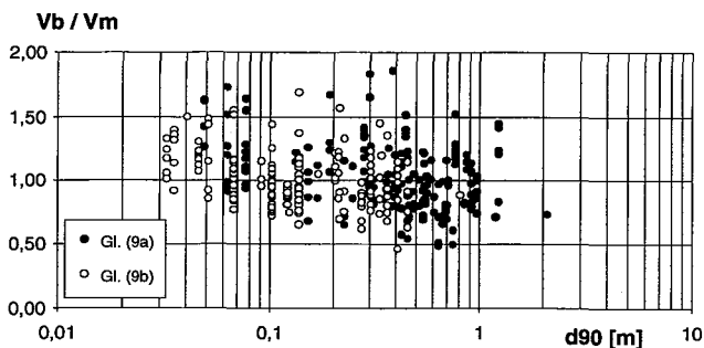
Bild 5. Verhältnis von berechneter zu gemessener Fließgeschwindigkeit, V_b/V_m , in Abhängigkeit der charakteristischen Korngröße d_{90} . Die Gleichung (9a) für steilere Gefälle ( J \geq 0,008 ) zeigt eine leichte Tendenz zur Überschätzung der Geschwindigkeit bei kleinen d_{90} .
