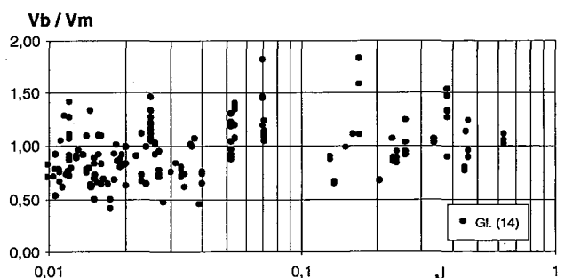
Bild 9. Verhältnis von berechneter zu gemessener Fließgeschwindigkeit, V_b/V_m , in Abhängigkeit des Gerinnegefälles J für Gleichung (14). Für die Daten mit Gefällen J \geq 5\% besteht die beste Übereinstimmung.
