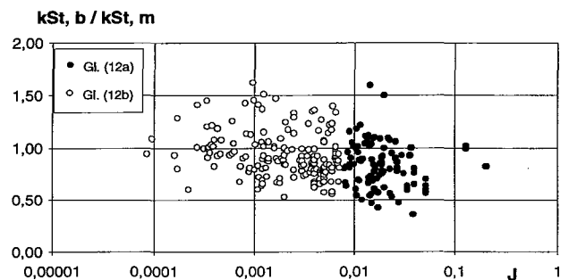
Bild 7. Verhältnis von berechnetem zu gemessenem Strickler -Wert, k_{St,b}/k_{St,m} , in Abhängigkeit des Gerinnegefälles J für die Gleichungen (12). Vor allem für den steileren Gefällsbereich ( J \geq 0,008 ) ergibt sich eine leichte, systematische Unterschätzung nach Gleichung (12a).
