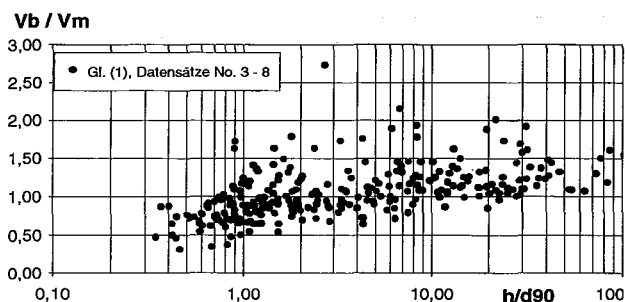
Bild 10: Verhältnis von berechneter zu gemessener Fließgeschwindigkeit, V_b/V_m , in Abhängigkeit der relativen Abflusstiefe h/d_{90} für Gleichung (1).
