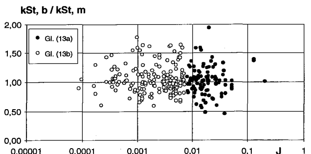
Bild 8. Verhältnis von berechnetem zu gemessenem Strickler -Wert, k_{St,b}/k_{St,m} , in Abhängigkeit des Gerinnegefälles J für die Gleichungen (13).
