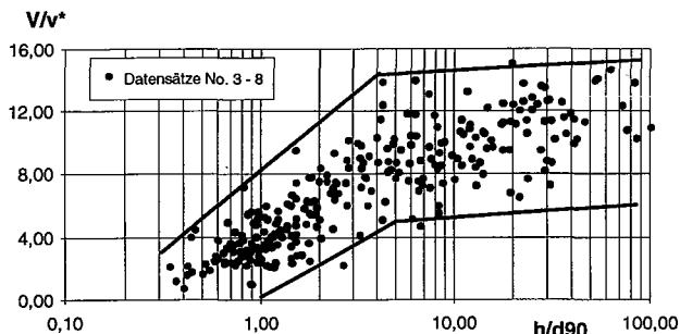
Bild 3. Der Kehrwert des Darcy-Weisbach-Reibungsbeiwertes, 1/v^* in Abhängigkeit der relativen Abflusstiefe h/d_{90} . Zur Verdeutlichung des generellen Verlaufs sind die Umhüllenden approximativ eingezeichnet. Im Bereich h/d_{90} zwischen 3 und 5 zeigt sich ein Knick in der Beziehung zwischen 1/v^* und h/d_{90} .
