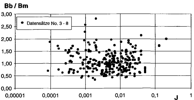
Bild 6. Verhältnis von berechneter zu gemessener (mittlerer) Gerinnebreite, B_b/B_m , in Abhängigkeit des Gerinnegefälles J .
