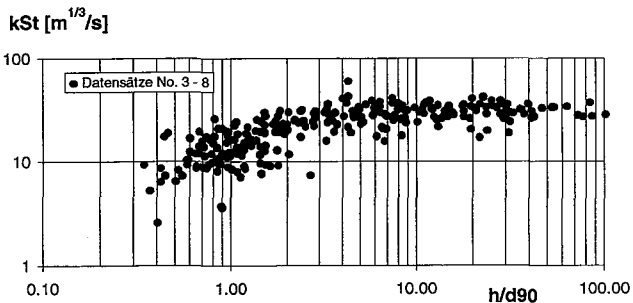
Bild 2. Strickler-Wert k_{St} in Abhängigkeit der relativen Abflusstiefe h/d_{90} . Für Werte h/d_{90} kleiner als etwa 3 bis 4 nimmt k_{St} deutlich ab.
